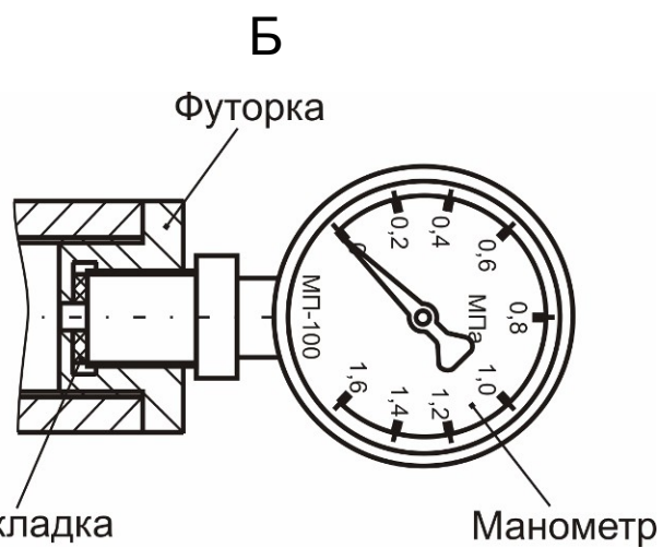
Рисунок 4.1 – Общий вид
